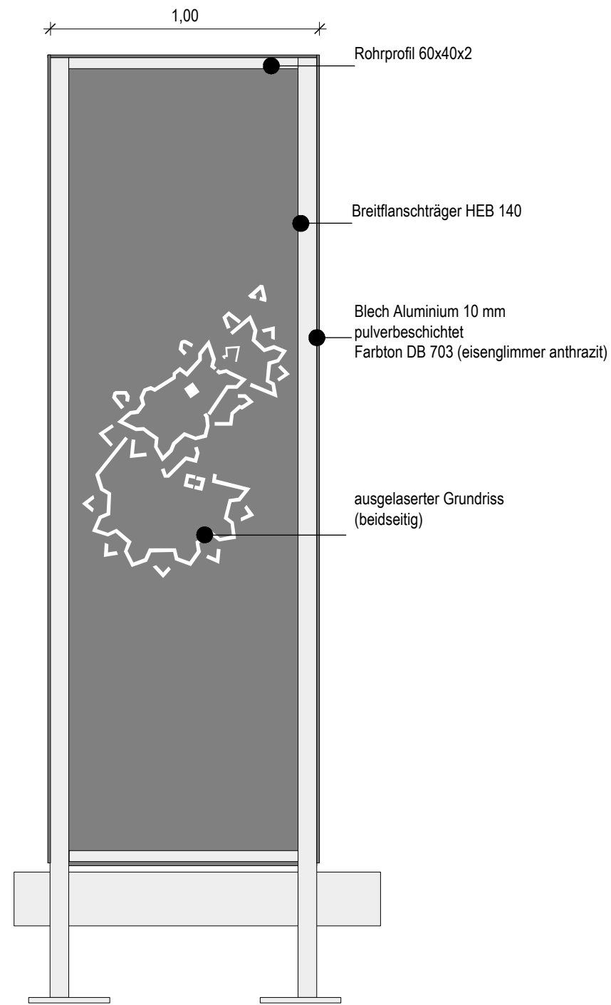
Konstruktionsprinzip 1 : 20
